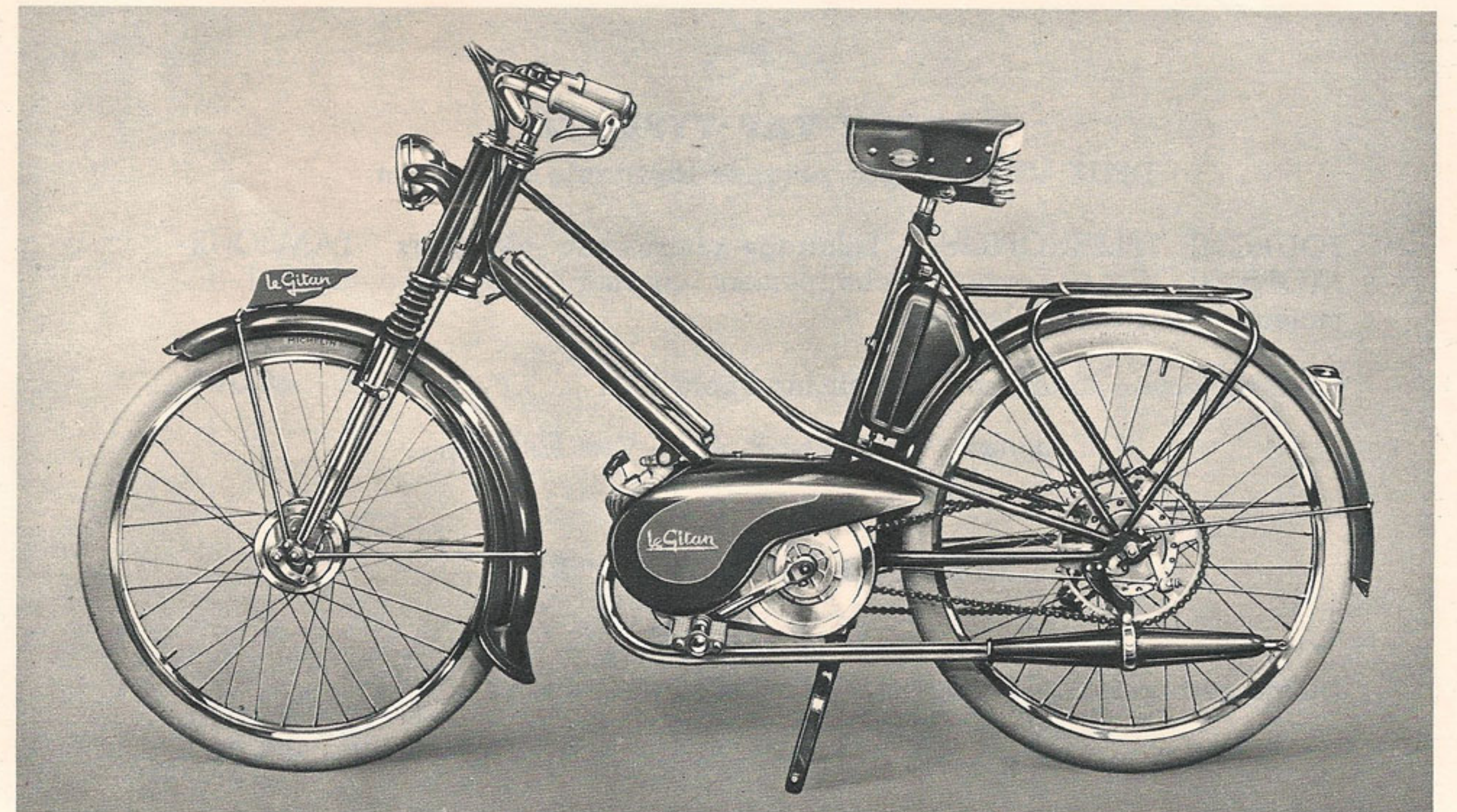
MODÈLE LUXE FOURCHE TÉLESCOPIQUE - Réservoir arrière - Moyeux tambour Monobloc - Eclairage phare-code - Avertisseur électrique. Tuyau d'échappement chromé. Couleurs : Noir, Bleu R. A. F., Vert Fougère, Gris Bleuté.
