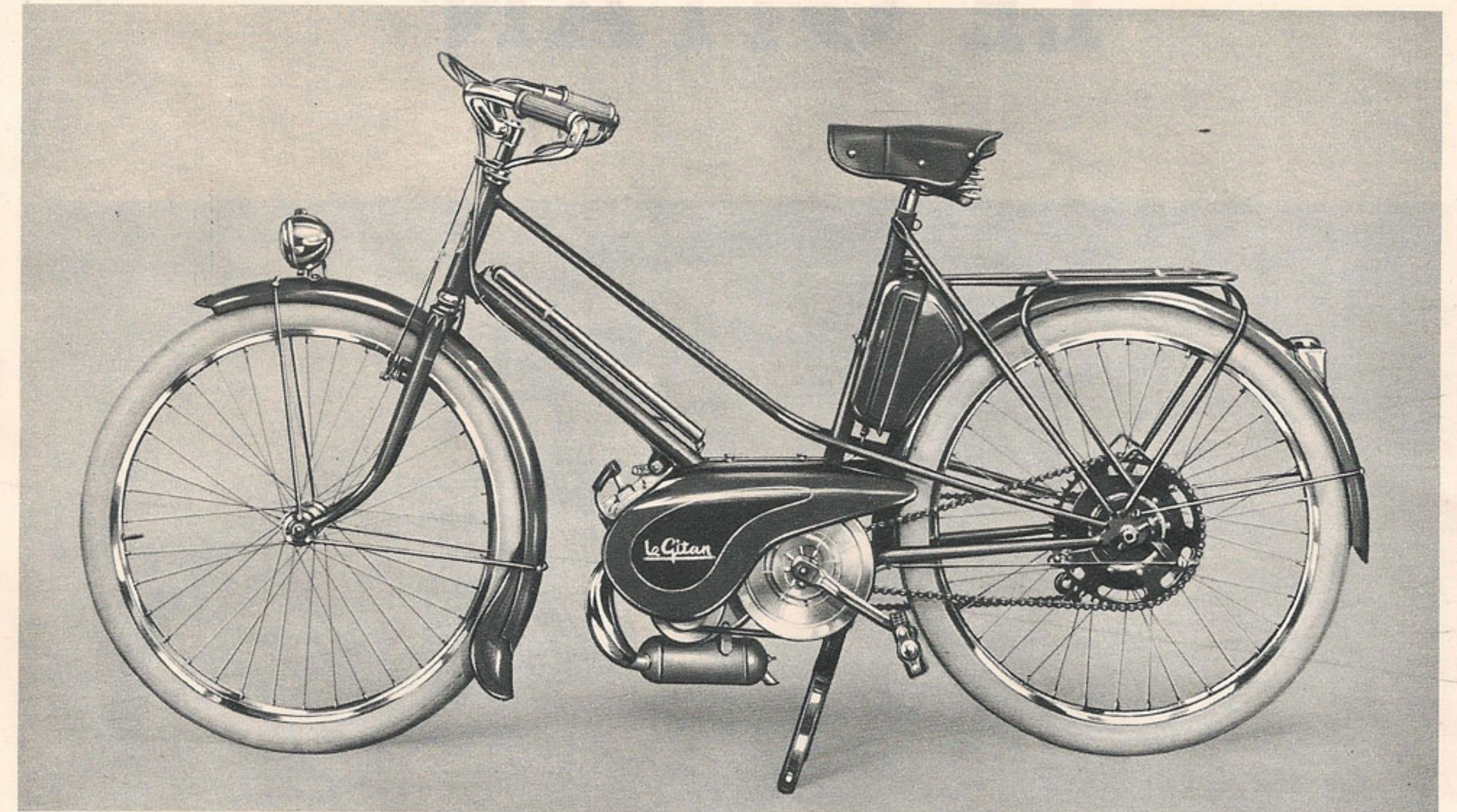
MODÈLE STANDARD - Fourche renforcée - Réservoir arrière - Moteur VAP ou MISTRAL à embrayage automatique (sur demande pour Mistral avec embrayage à main sans supplément). - Bleu R. A. F. N° 16 bis , moteur MISTRAL 39.800 N° 22, moteur VAP 55 41.100
