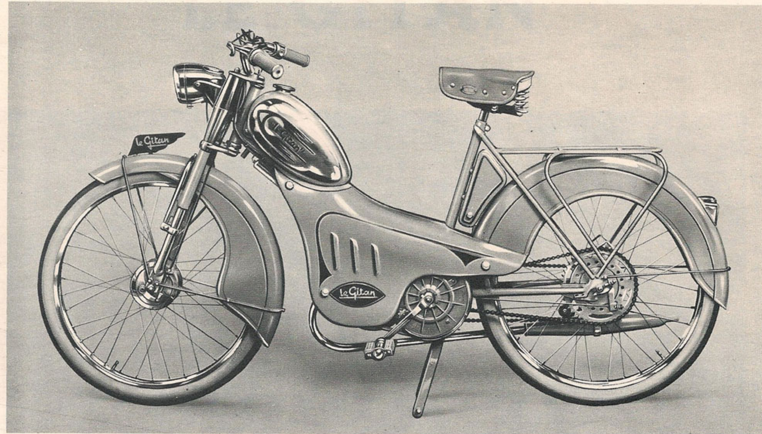
NOUVEAU MODÈLE CARÈNE - Réservoir semi-chromé 5 litres - Moyeux tambour Monobloc - Projecteur laiton phare-code avec compteur - Pneus bicolores - Avertisseur électrique - Tuyau d'échappement chromé. Couleurs : Vert Fougère, Gris Bleuté.
