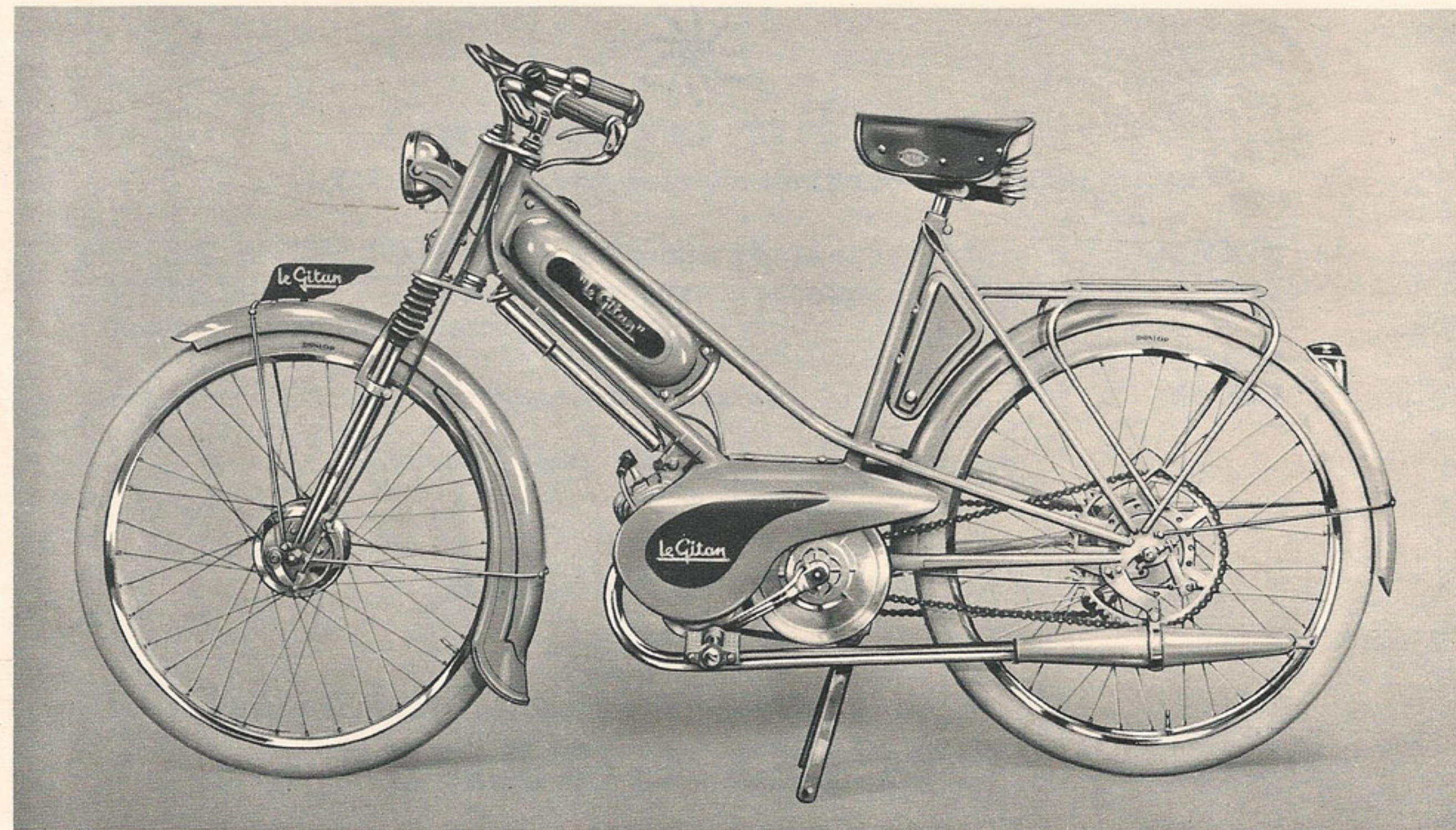
NOUVEAU MODÈLE LUXE - Réservoir avant 3 litres - Moyeux tambour Monobloc - Eclairage phare-code - Avertisseur électrique - Tuyau d'échappement chromé. Couleurs : Noir, Bleu R. A. F., Vert Fougère, Gris Bleuté.
