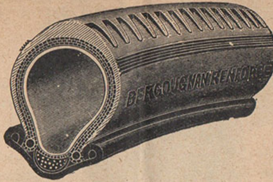
ENVELOPPE « BERGOUGNAN » « LE GAULOIS » Renforcée, à tringles, « sculptée », à triple entoilage.
