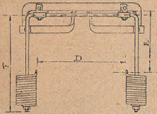
Croquis de la selle " Terry ". Suspension en traction.
