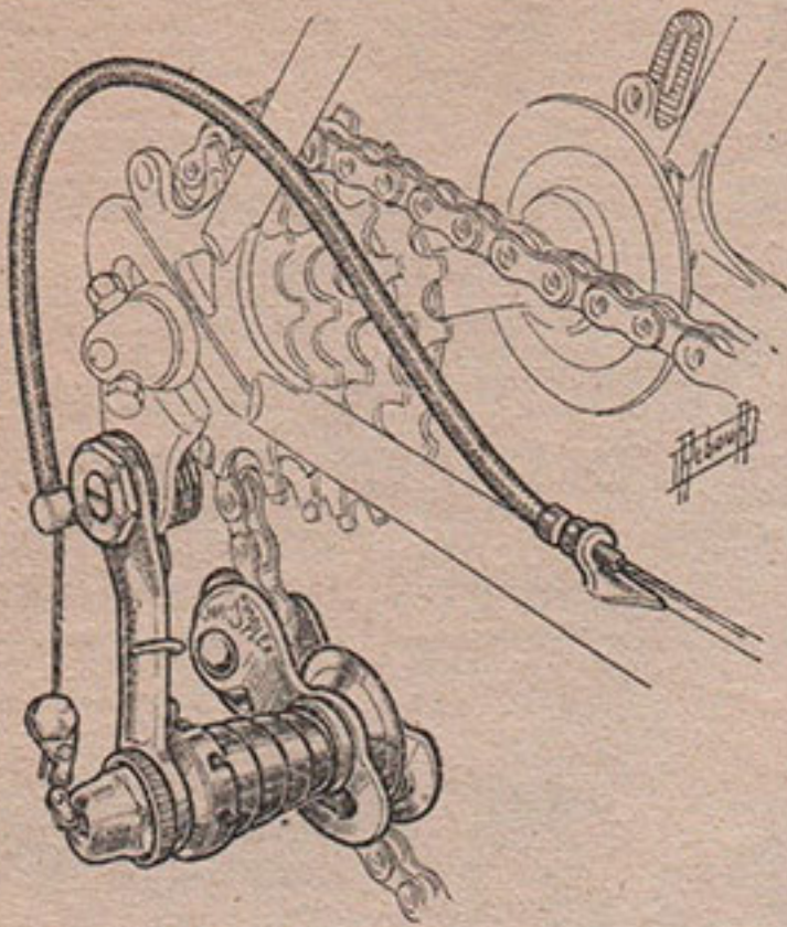
SIMPLEX Type « Tour de France » 4111 3 vitesses la pièce 650 » 4112 4 — — — 660 »
