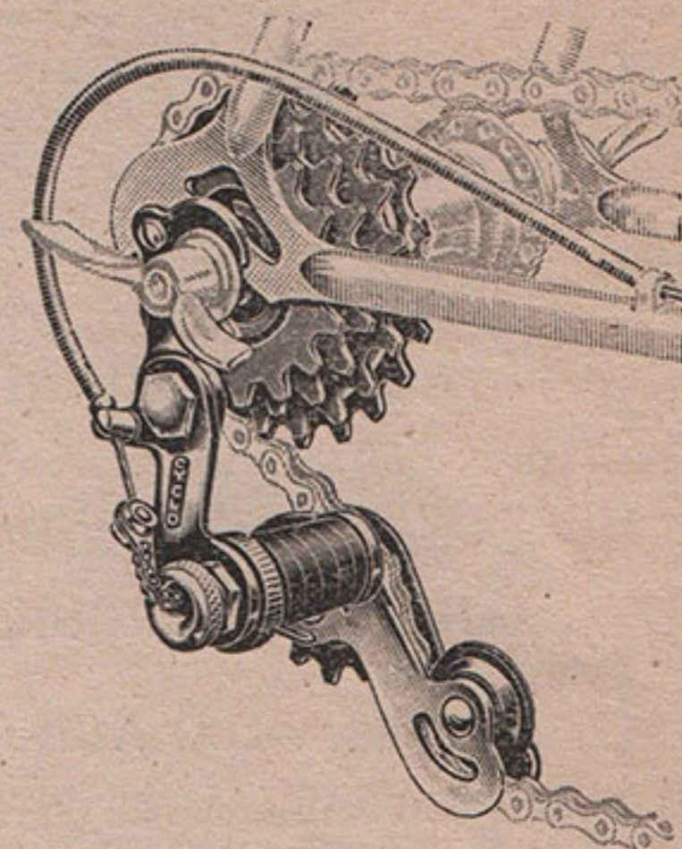
4103 Cyclo course Commande Monocâble 4 vitesses Prix : 600 »
