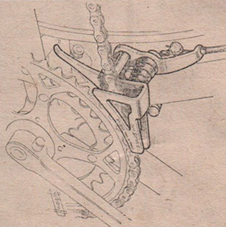
SIMPLEX DE PÉDALIER TYPE 39 pour TANDEM à collier 4125 la pièce ..... Prix 725 »
