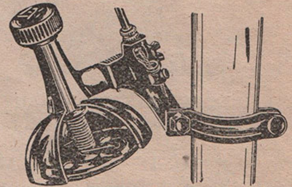
AVERTISSEUR ROTATIF E. M. Calotte acier chromé Commande au guidon Modèle Cycle 5307 Prix ..... 360 » Modèle renforcé Cyclomoteur 5308 Prix ..... 377 »
