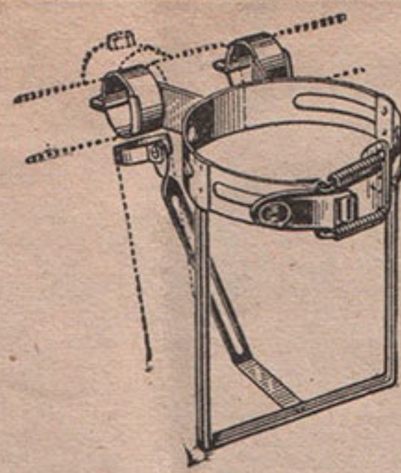
Pour 1 bidon sur guidon 5282 Prix 130 »
