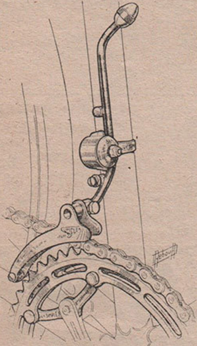
SIMPLEX DE PÉDALIER Type « Compétition » 4123 la pièce ..... 550 »
