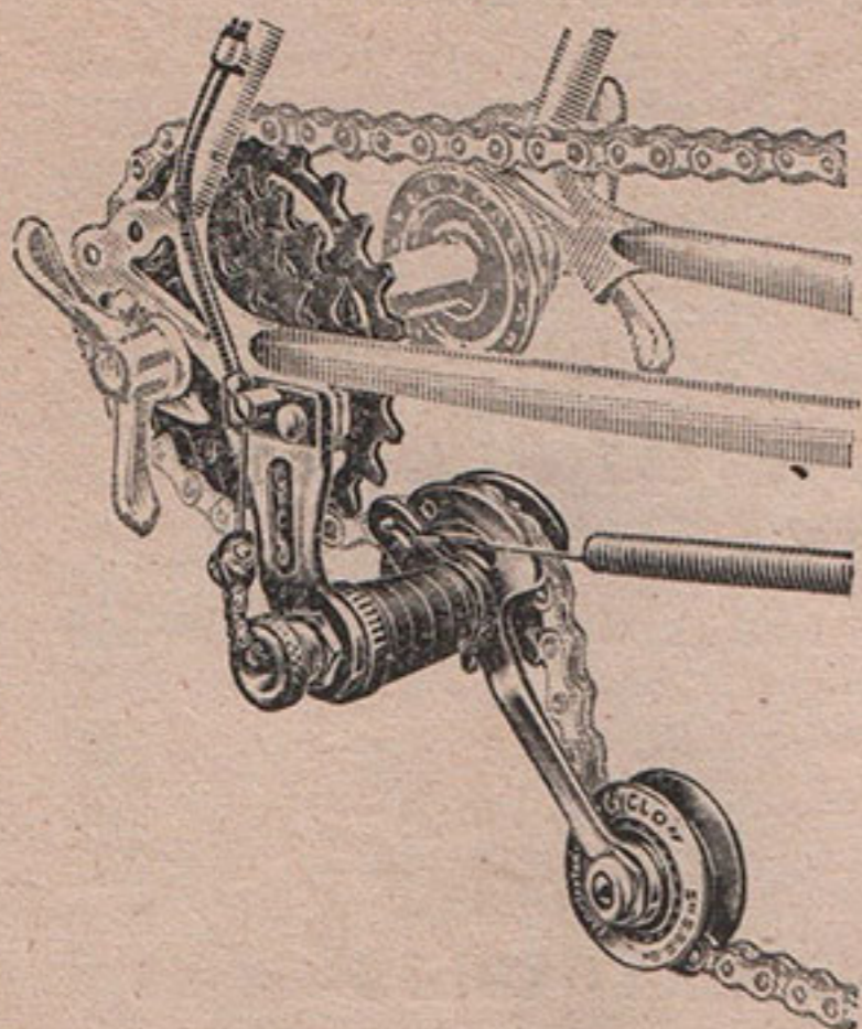
4102 Cyclo route Commande Monocâble 3 ou 4 vitesses Prix : 600 »
