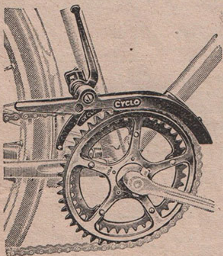
DÉRAILLEUR DE PÉDALIER CYCLO Commande rigide
