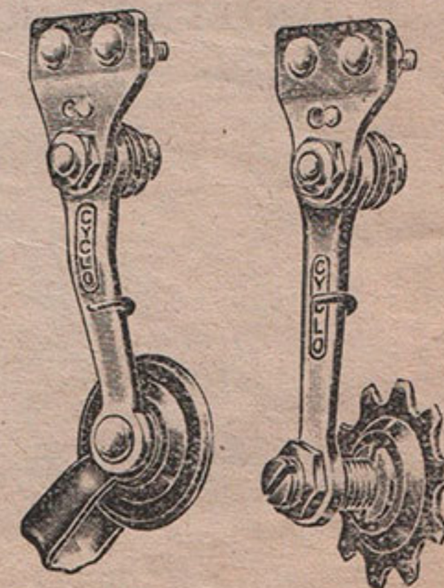
TENDEURS DE CHAÎNE Pour cyclomoteurs 4149 A galet .... 160 » 4150 A pignon .. 180 » Le modèle à pignon est réglable
