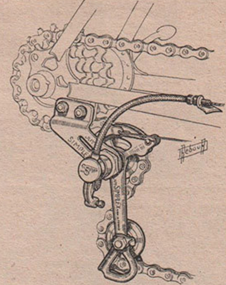
SIMPLEX Type « Grand Tourisme » 4113 3 vitesses la pièce 650 » 4114 4 — — — 660 »
