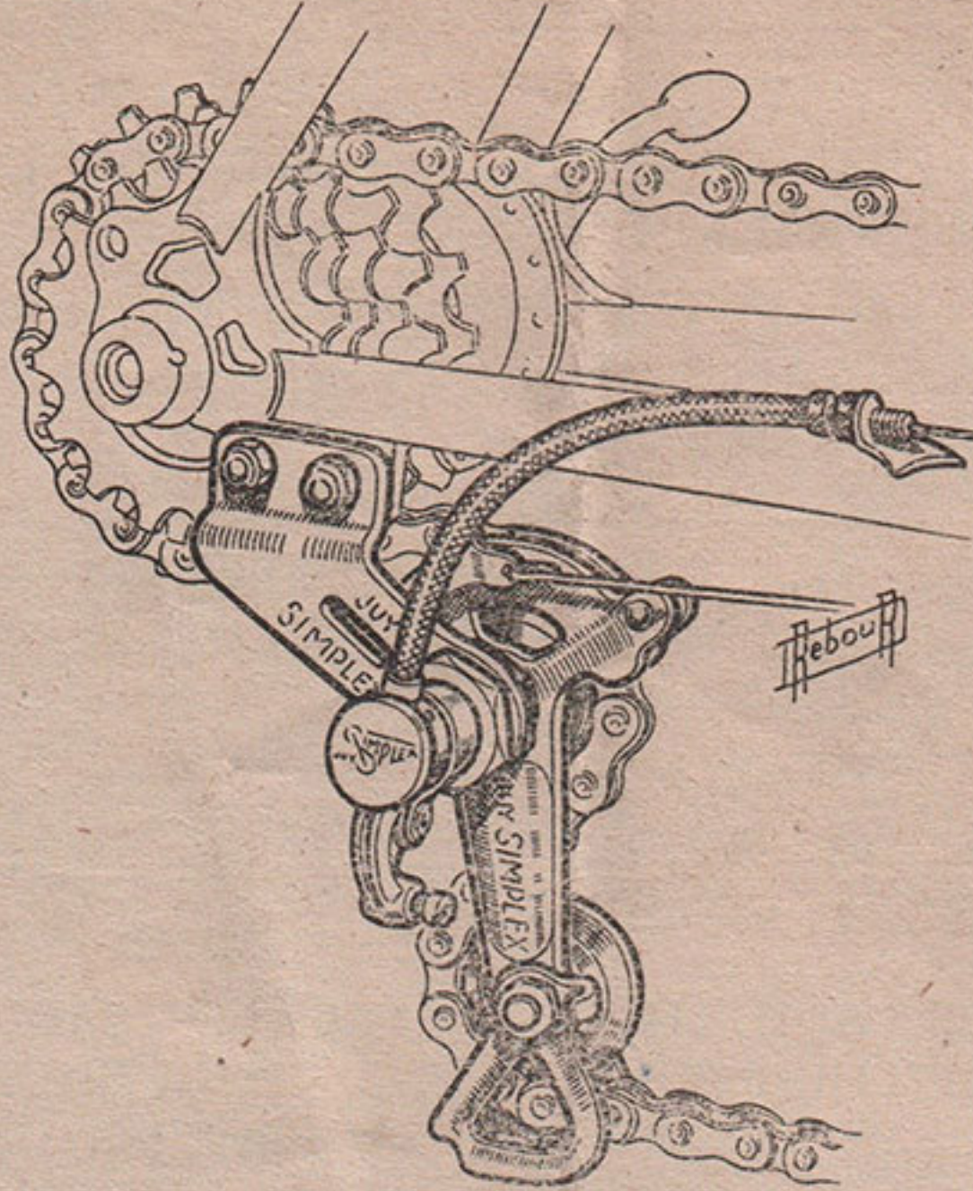
SIMPLEX TYPE « RIGIDEX » Modèle renforcé 4115 3 vitesses ..... la pièce 670 » 4116 4 — ..... — 680 »
