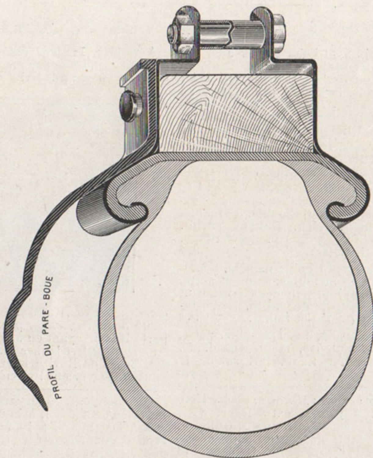
COUPE DU PARE-BOUE GARCHEY
