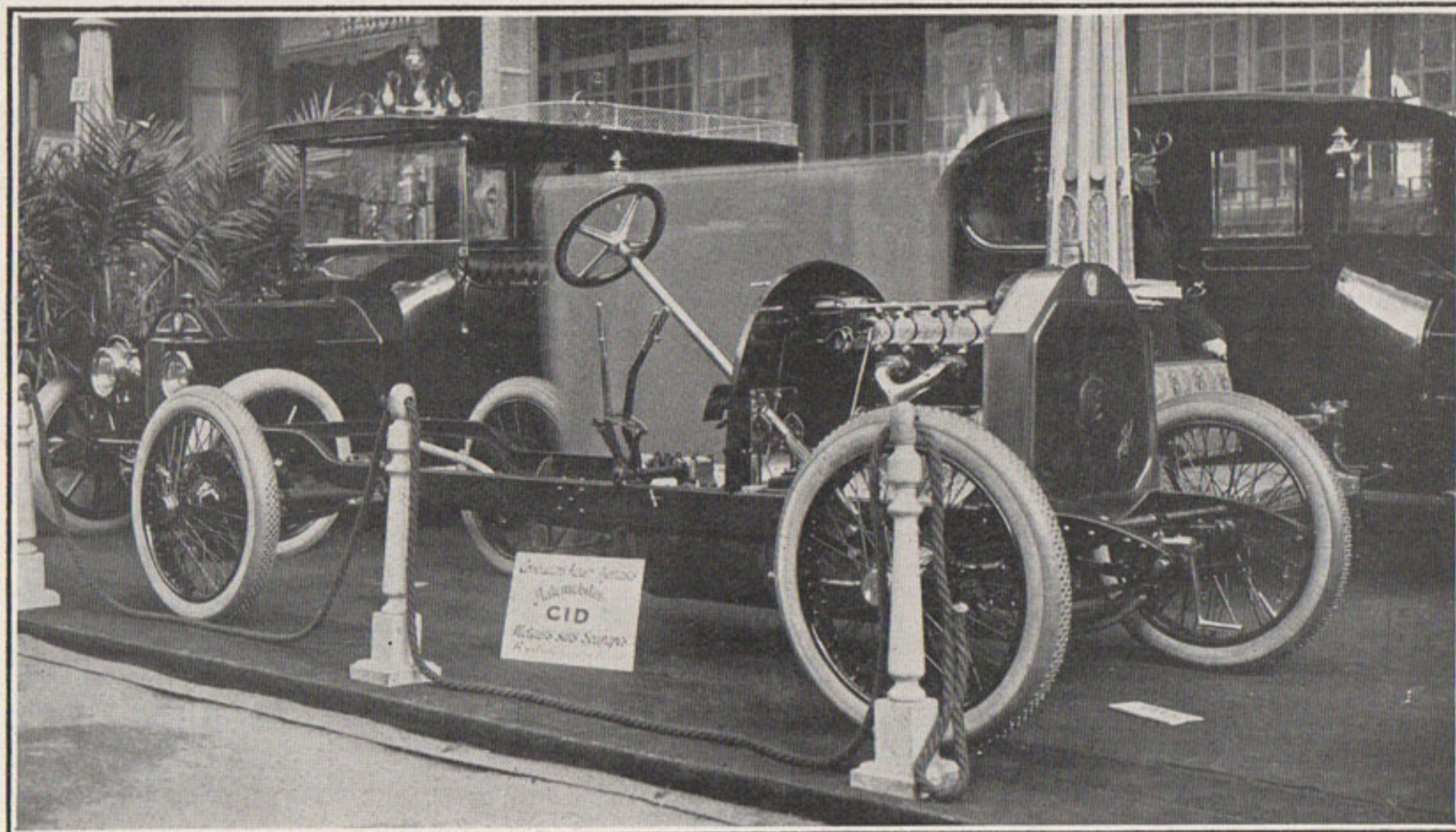
CHASSIS 12 HP C. I. D. MOTEUR 4 CYLINDRES SANS SOUPAPES 75×120
