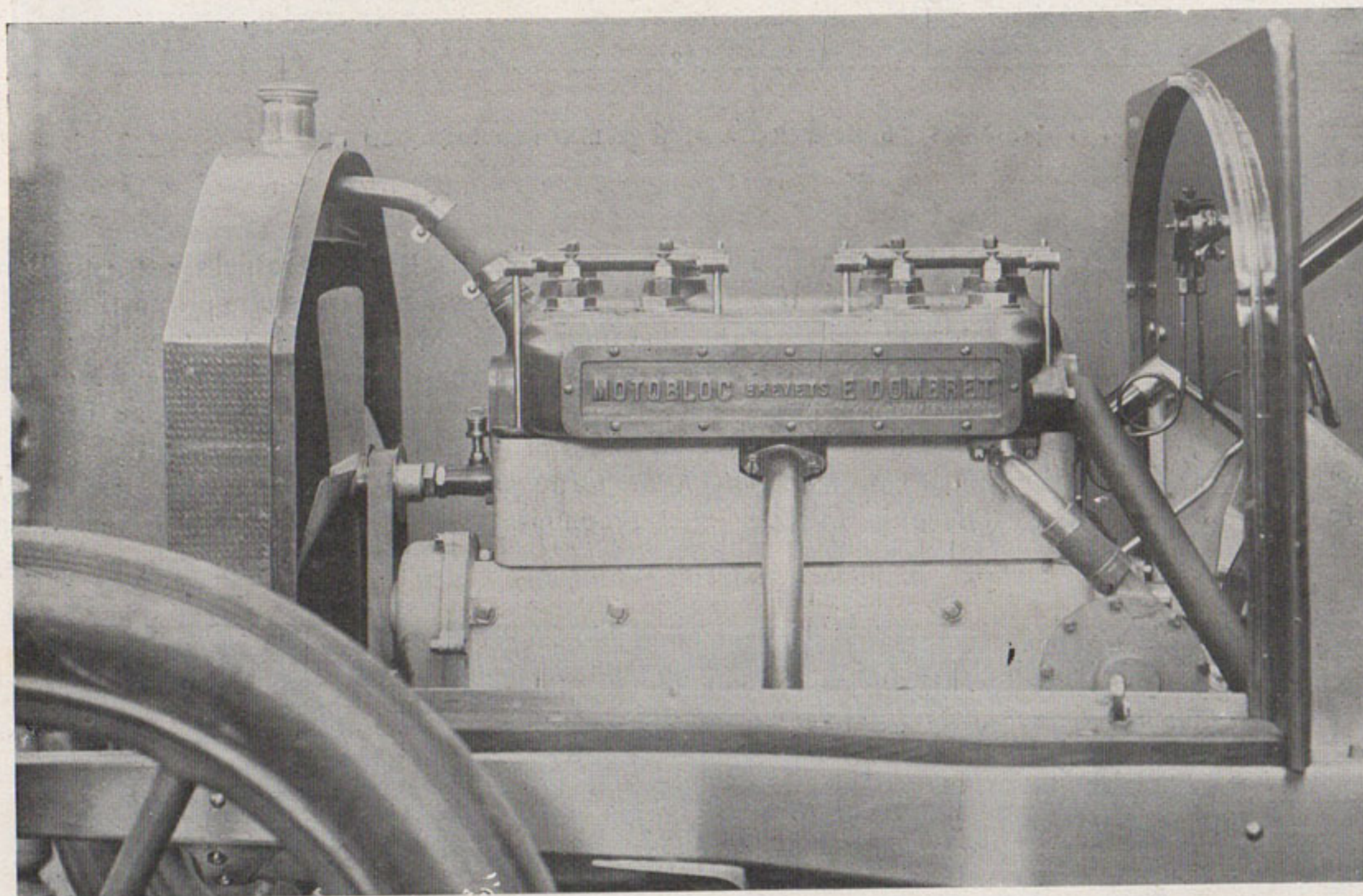
BLOC-MOTEUR E. DOMBRET 4 CYLINDRES 1913
