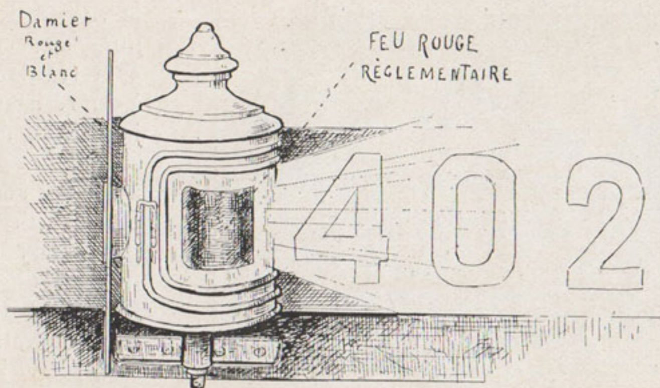
POSITION DE L'AUTOMATIC-PROTECTOR, LA VOITURE EN MARCHÉ
